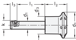
销 Ø 6 / 8 单侧滚珠固定
